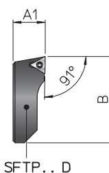
SFTP... D
