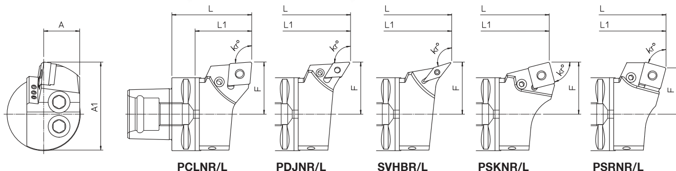
PCLNR/L
