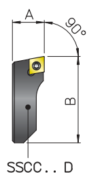
SSCC... D
